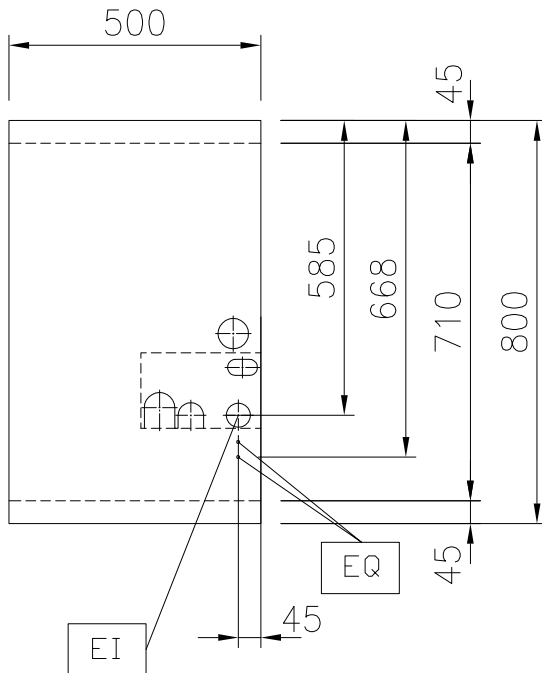
Boven aanzicht
